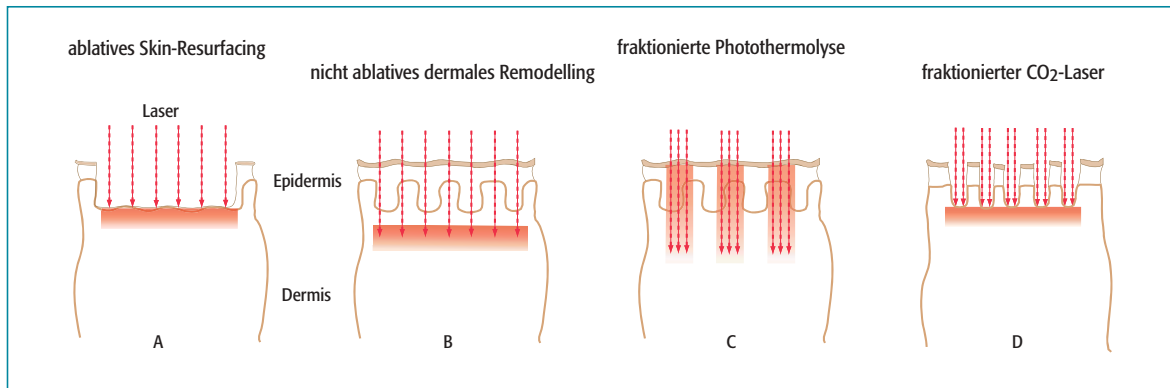
Abbildung 1: Konzeptioneller Methodenvergleich
